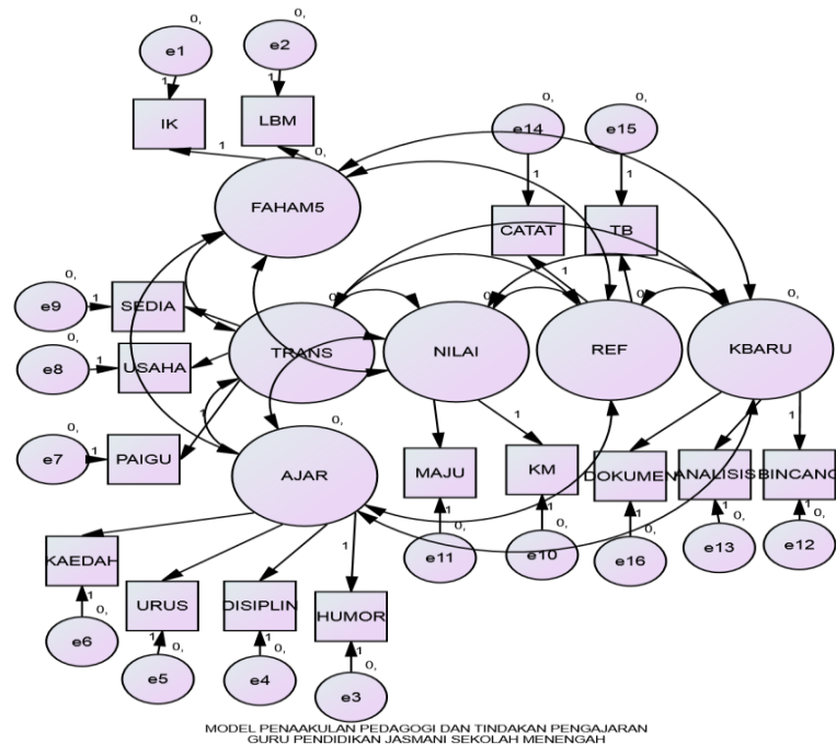
Rajah 2. Model Pengukuran Penuh (Summited)
