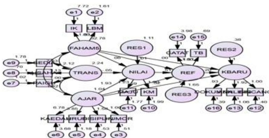
Rajah 3. Model Pengukuran Analisis
